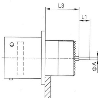
receptacle (RF27466)
