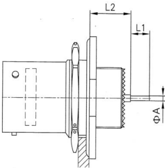
receptacle (RF27468)
